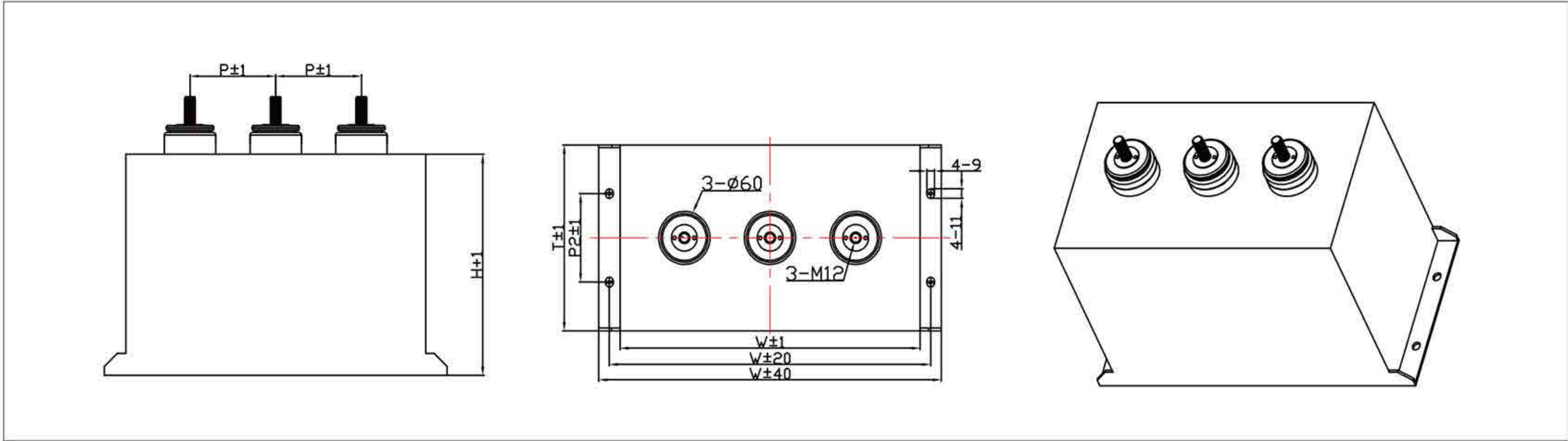
外形图 The contour map
