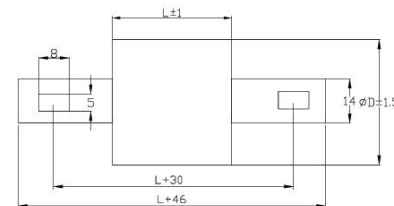
D0引出方式 D0 lead-out method
